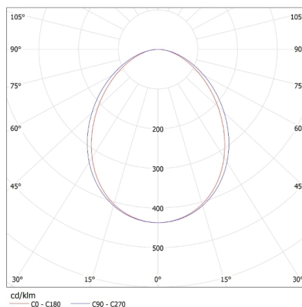
KANLUX S.A. (kat 29419) AL 23W-840-MAT-B-NT / LDC (Polar)
