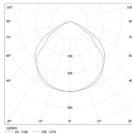
MILED0 (kat 31150) GRUN V2 LED-10-B / LDC (Polar)
