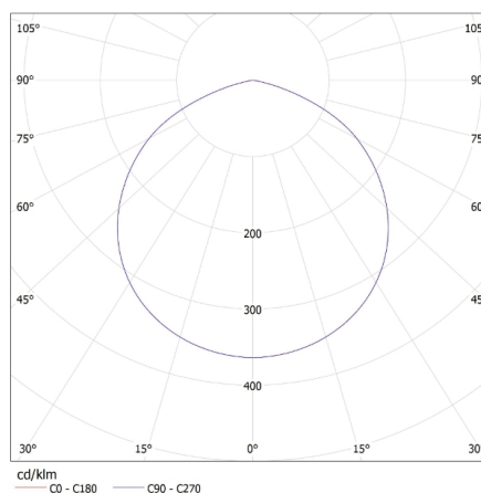
MILED0 (kat 31152) GRUN V2 LED-30-B / LDC (Polar)
