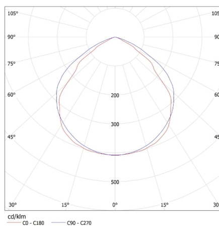
MILEDO (kat 31154) GRUN V2 LED-10-B-SE / LDC (Polar)
