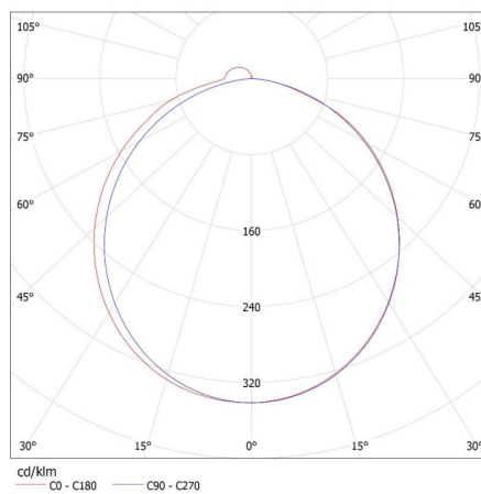
KANLUX S.A. (kat 26680) ASTEN LED IP44-8W-NW / Krzywa rozsyłu światła (biegunowo)
