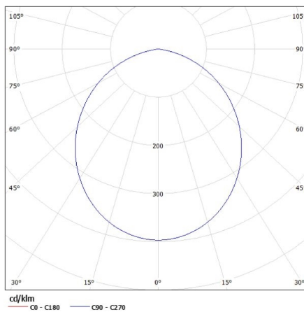
KANLUX S.A. (kat 23520) IMBER LED NW / Krzywa rozsytu światła (biegunowo)
