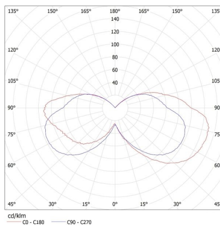
KANLUX S.A. (kat 23101) SOLA LED / Krzywa rozsytu światła (biegunowo)
