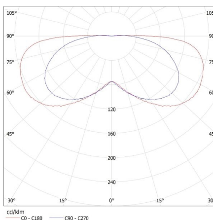
KANLUX S.A. (kat 23105) TERRA MINI LED / Krzywa rozsytu światła (biegunowo)
