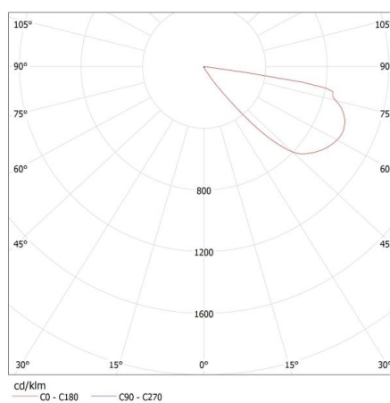
KANLUX S.A. (kat 22760) ONSTAR LED-GR / Krzywa rozsytu światła (biegunowo)
